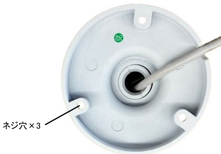
図3-2 カメラの固定
