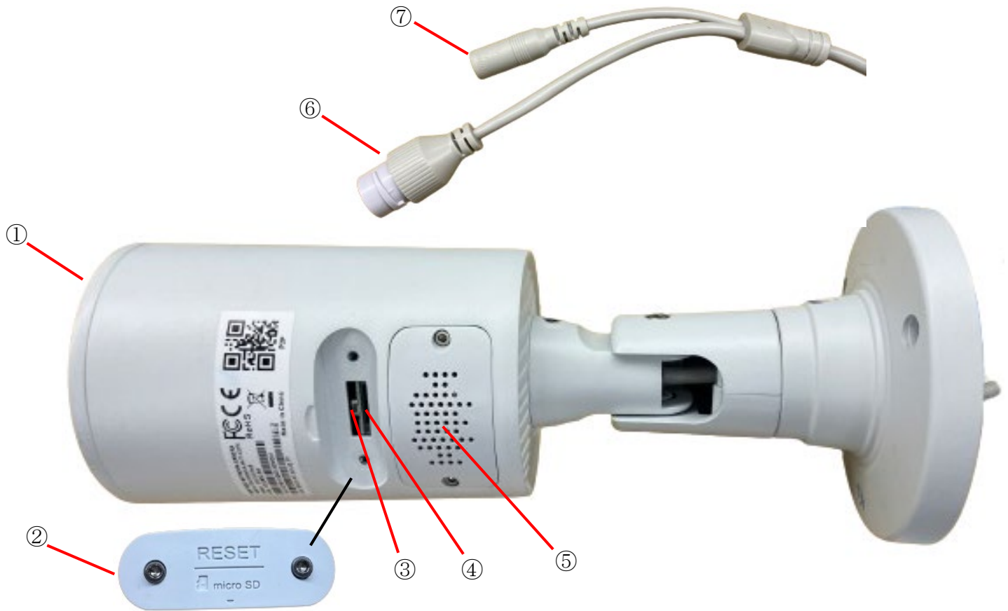
図2-1 外観図
